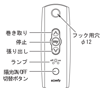
陽光センサー ON/OFF切替ボタン付
